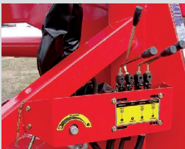
COMANDOS HIDRÁULICOS INDEPENDIENTES. VÁLVULA REGULADORA DE VELOCIDAD DE AVANCE.
